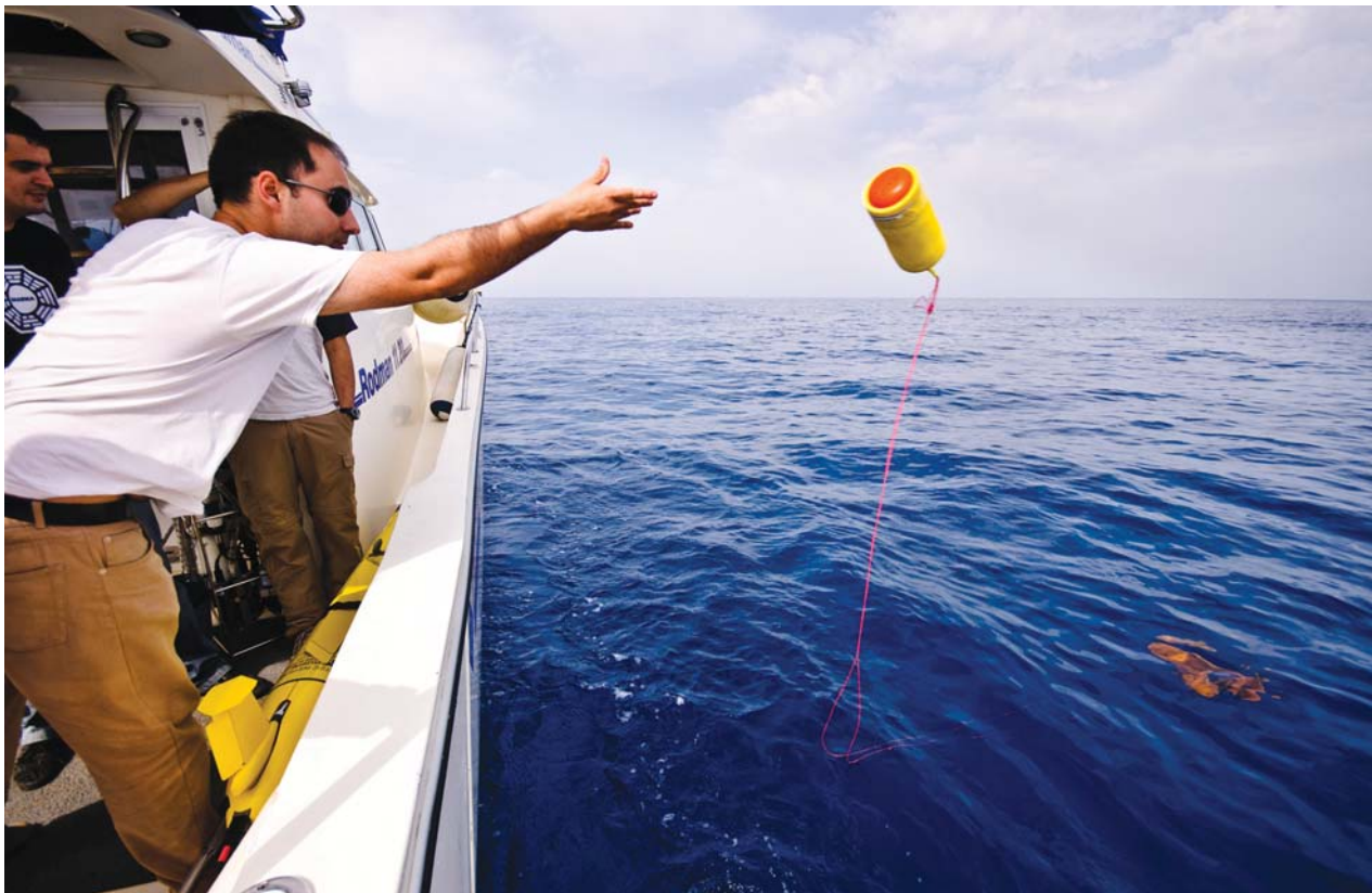
Boya Lagrangiana
